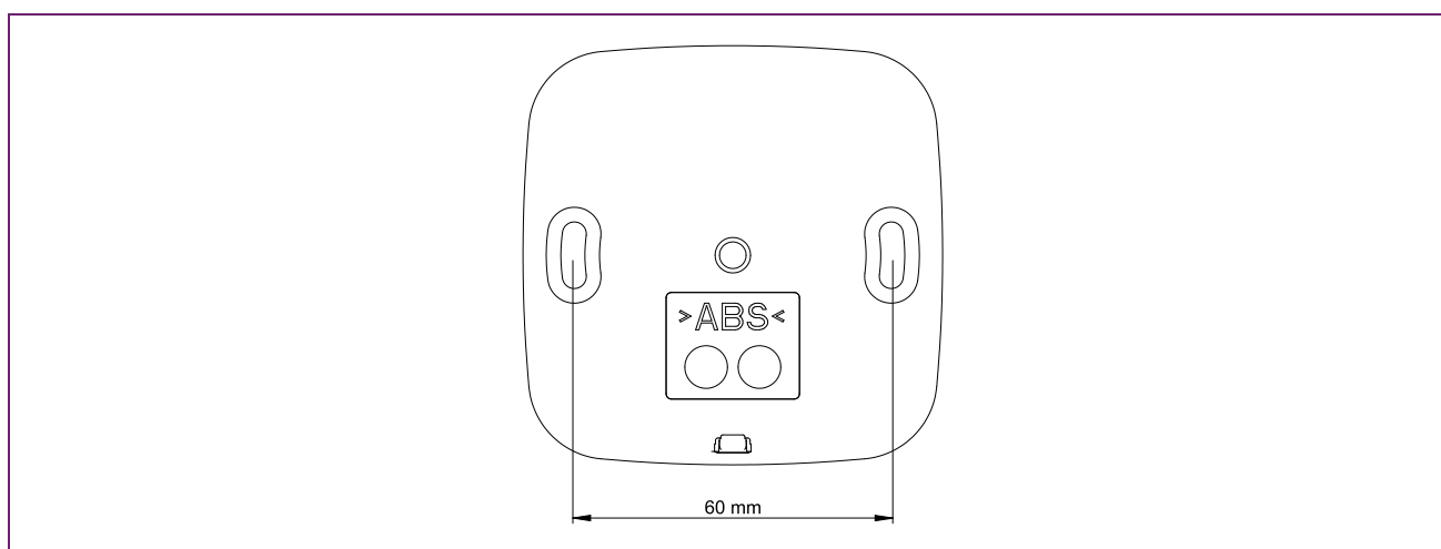
Abb. 1: Bohrbild
